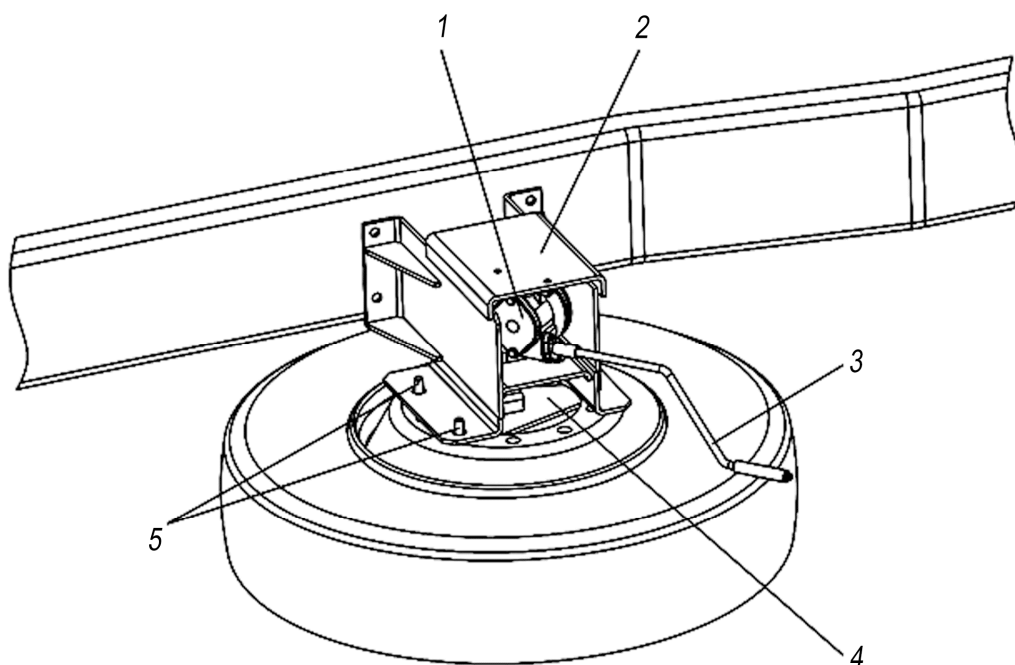
1-редуктор с тросом; 2-держатель запасного колеса; 3-рукоятка съемная; 4-плита крепления колеса; 5-гайки крепления колеса на держателе запасного колеса
