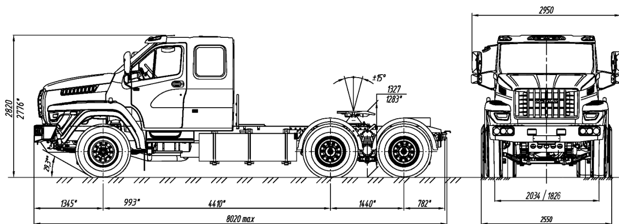
Рисунок 3.4 – Габаритные размеры седельного тягача Урал-7470-5511-01
