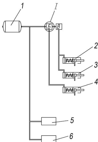
Рисунок 5.2.4 (б) - Электропневмоуправление агрегатами трансмиссии с двигателем ЯМЗ-653
