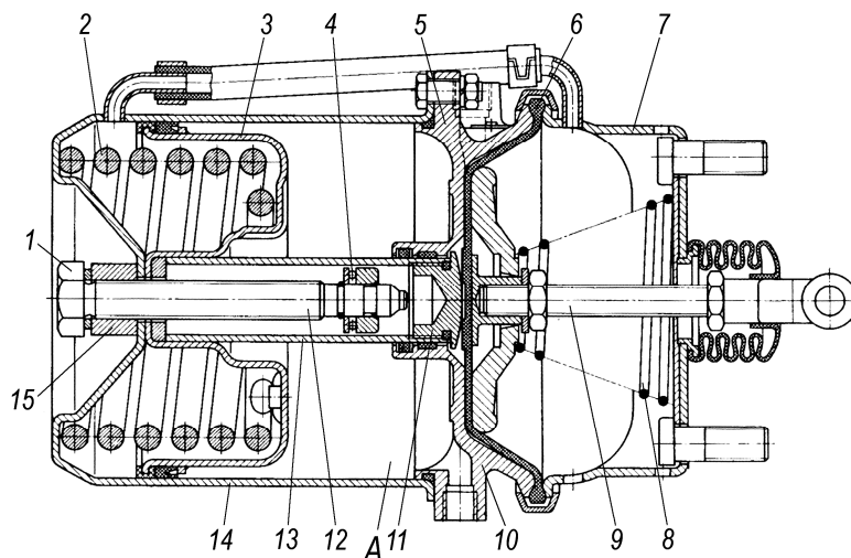
1-винт; 2-пружина силовая; 3-мембрана; 4-шарик; 5-диск; 6-диафрагма; 7-корпус тормозной камеры; 8-пружина возвратная; 9-шток тормозной камеры; 10-фланец; 11-втулка фиксирующая; 12-шток пружинного энергоаккумулятора; 13-толкатель; 14-корпус пружинного энергоаккумулятора; 15-втулка направляющая; А-полость
