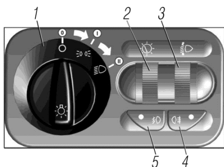
1-центральный переключатель света; 2-регулятор освещенности приборов; 3-регулятор корректора фар; 4-выключатель передних противотуманных фонарей*; 5-выключатель задних противотуманных фонарей
