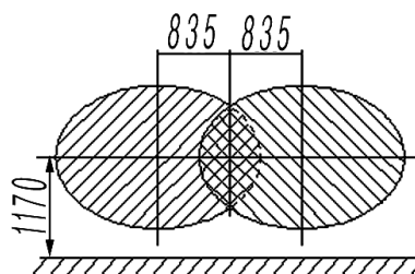
Рисунок 5.6.19 - Разметка экрана для регулировки фар дальнего света
