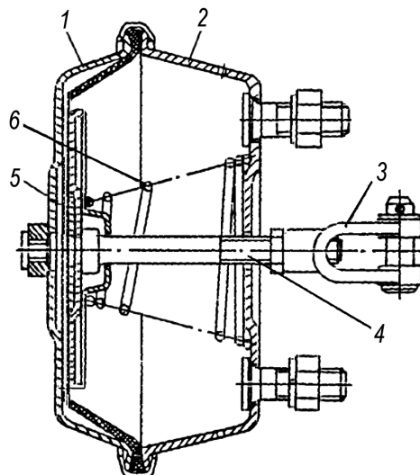
1-крышка; 2-корпус; 3-вилка; 4-шток с диском; 5-мембрана; 6-пружина возвратная
