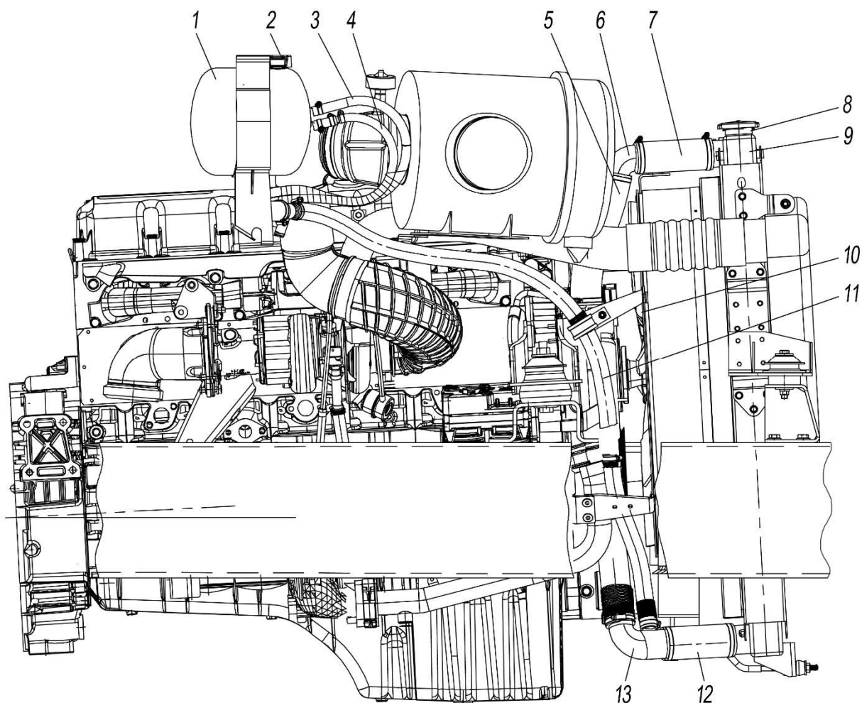
1-бачок расширительный; 2-пробка расширительного бачка; 3-рукав пароотводящий от радиатора; 4-рукав пароотводящий от двигателя; 5,7-рукав отводящий от двигателя; 6-патрубок водоподводящий; 8-горловина заливная радиатора; 9-блок радиаторов с кожухом; 10-вентиль; 11-трубопровод водоподводящий; 12-рукав подводящий к двигателю; 13-труба водоподводящая
