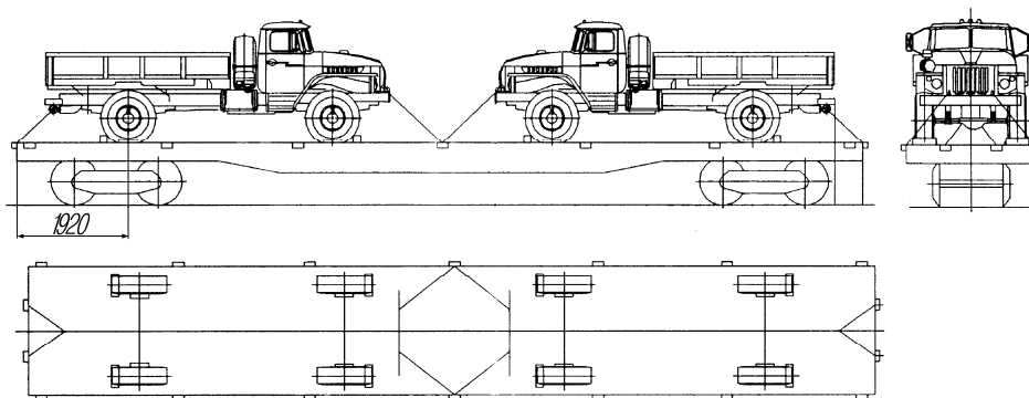
Рисунок 141- Схема погрузки и крепления автомобилей на четырехосной платформе (для автомобилей 4х4)
