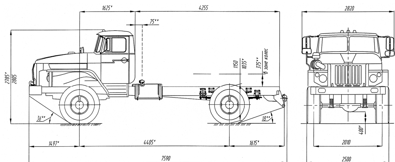
Рисунок 14 - Габаритные размеры шасси Урал- 43206-1151-61
