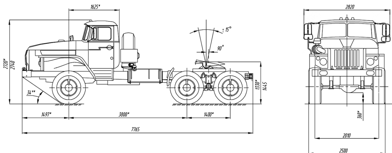
Рисунок 15 - Седельные тягачи Урал- 44202-0311- 60
