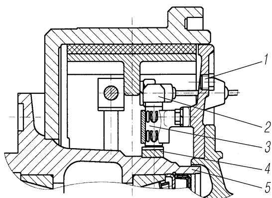
1-пробка; 2-датчик индуктивный; 3-втулка зажимная; 4-кольцо импульсное зубчатое; 5-ступица колеса
