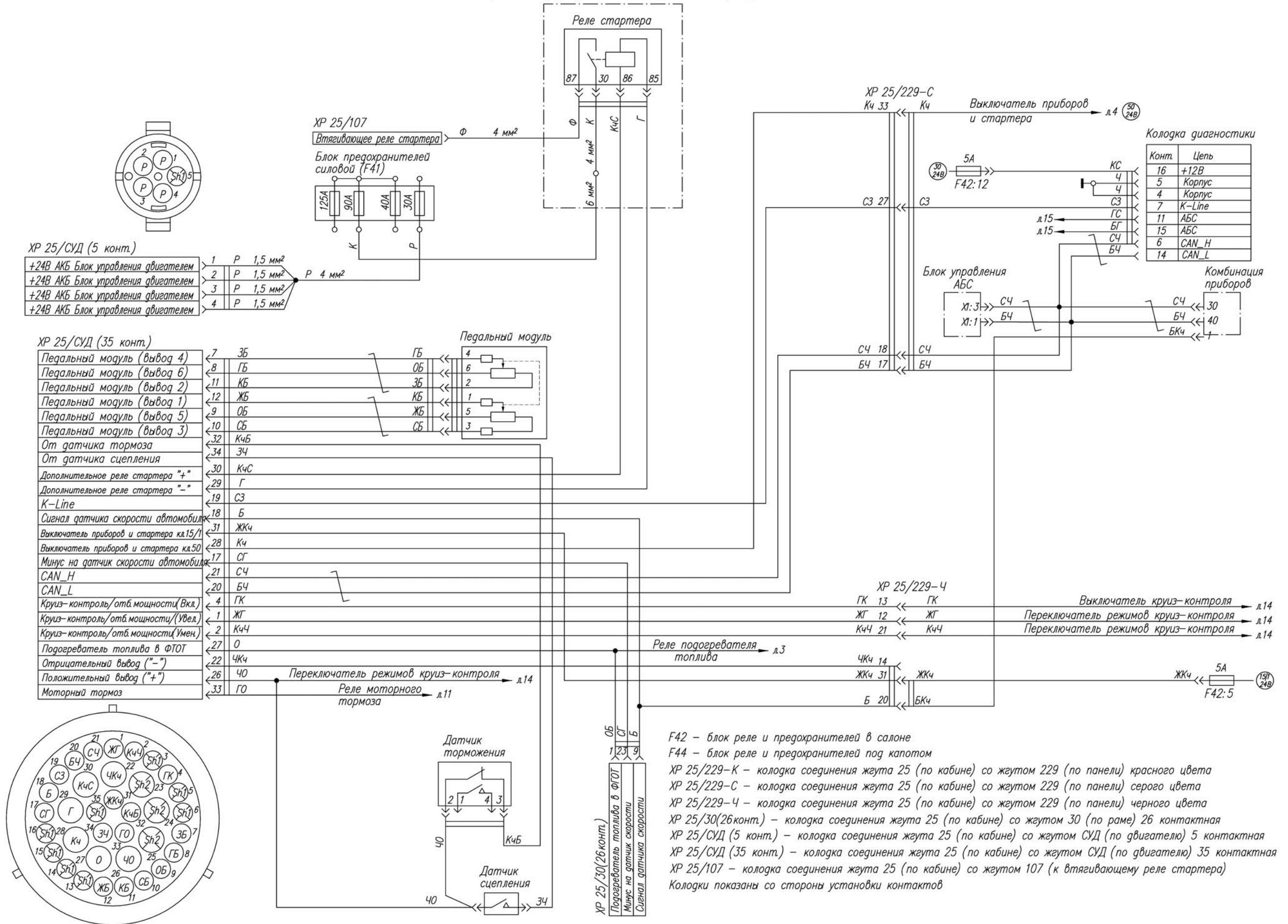
Рисунок 5.6.8 - Схема электрооборудования кабины
