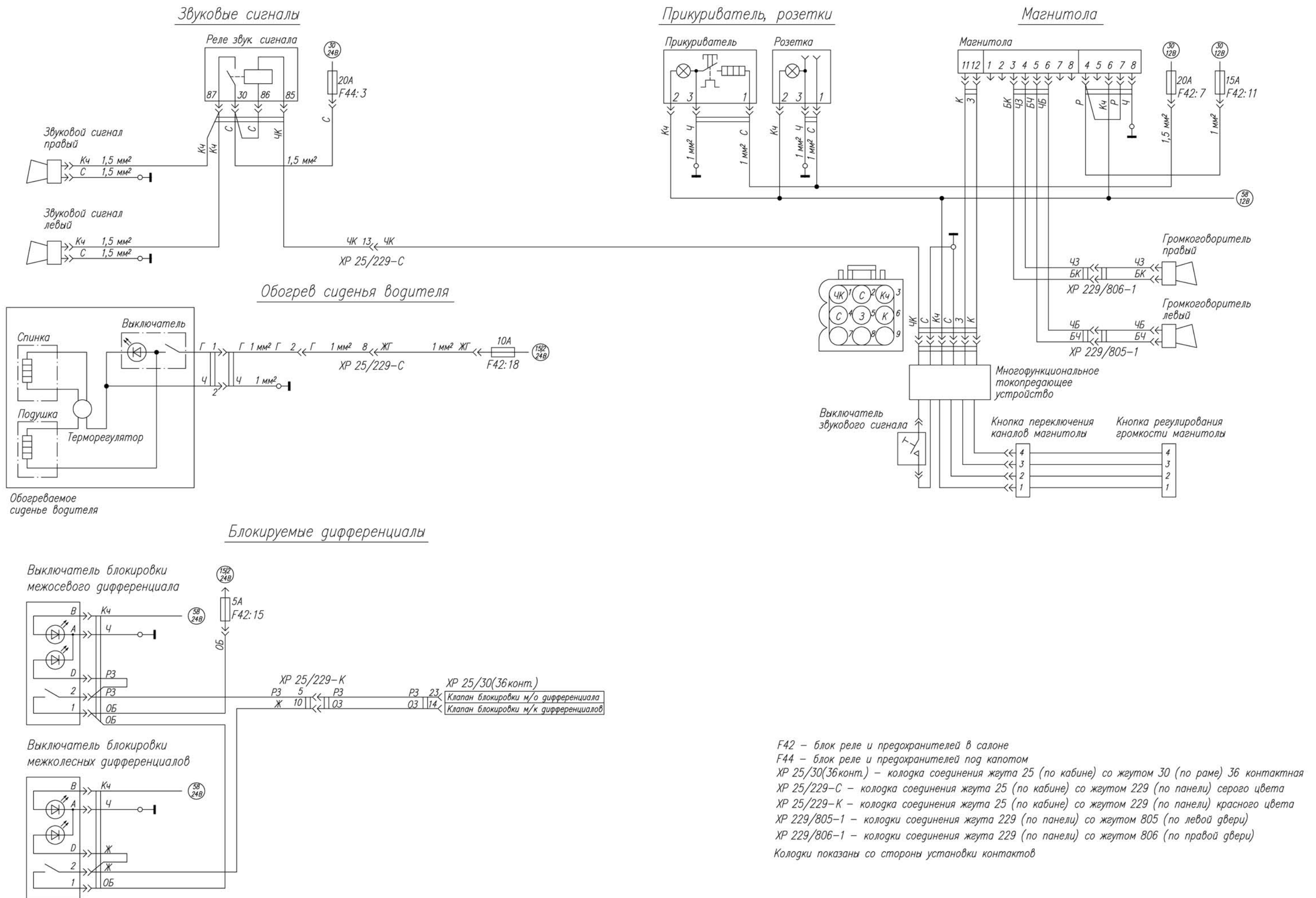
Рисунок 5.6.7 - Схема электрооборудования кабины
