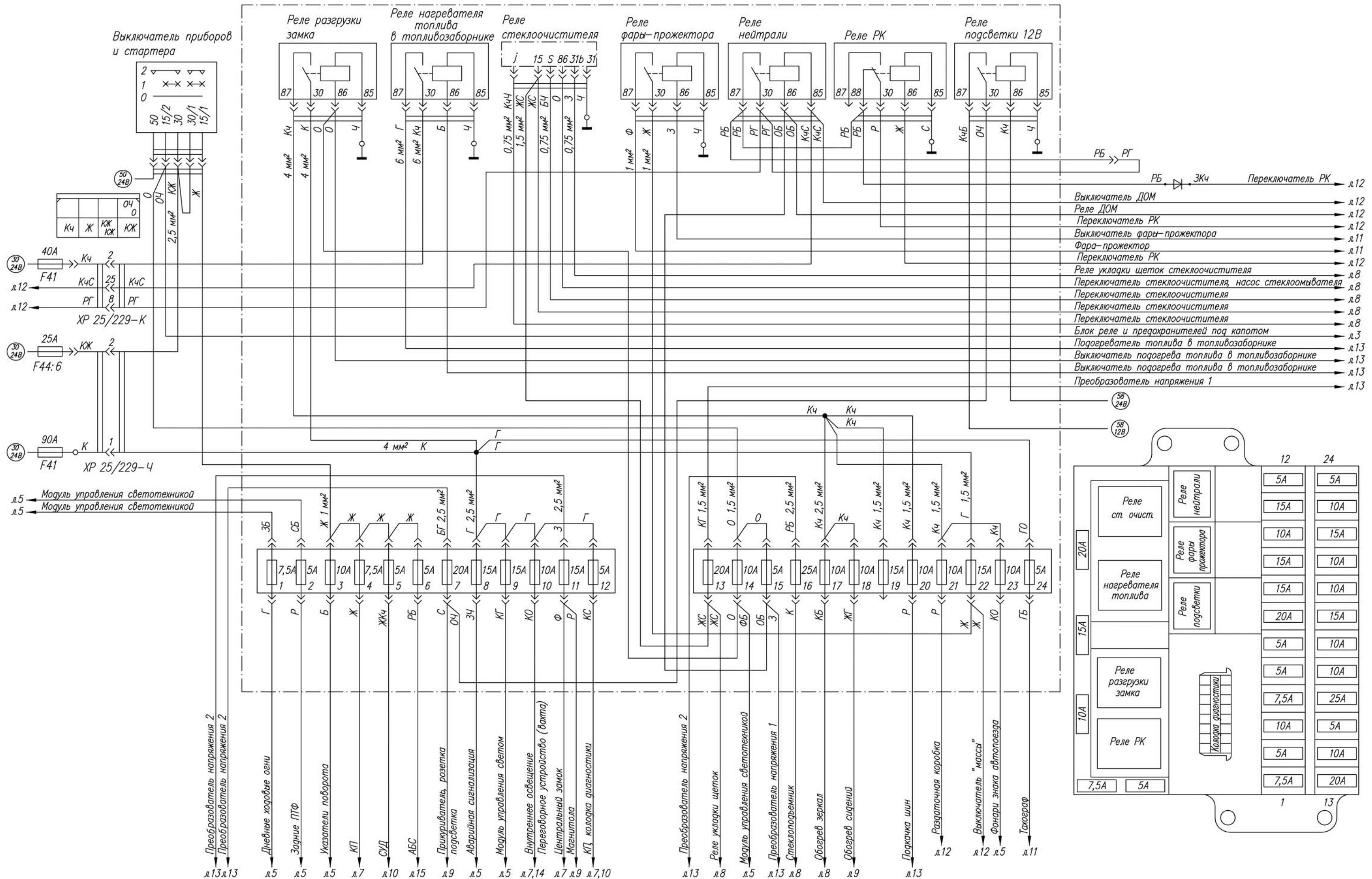
Рисунок 5.6.2 - Схема электрооборудования кабины
