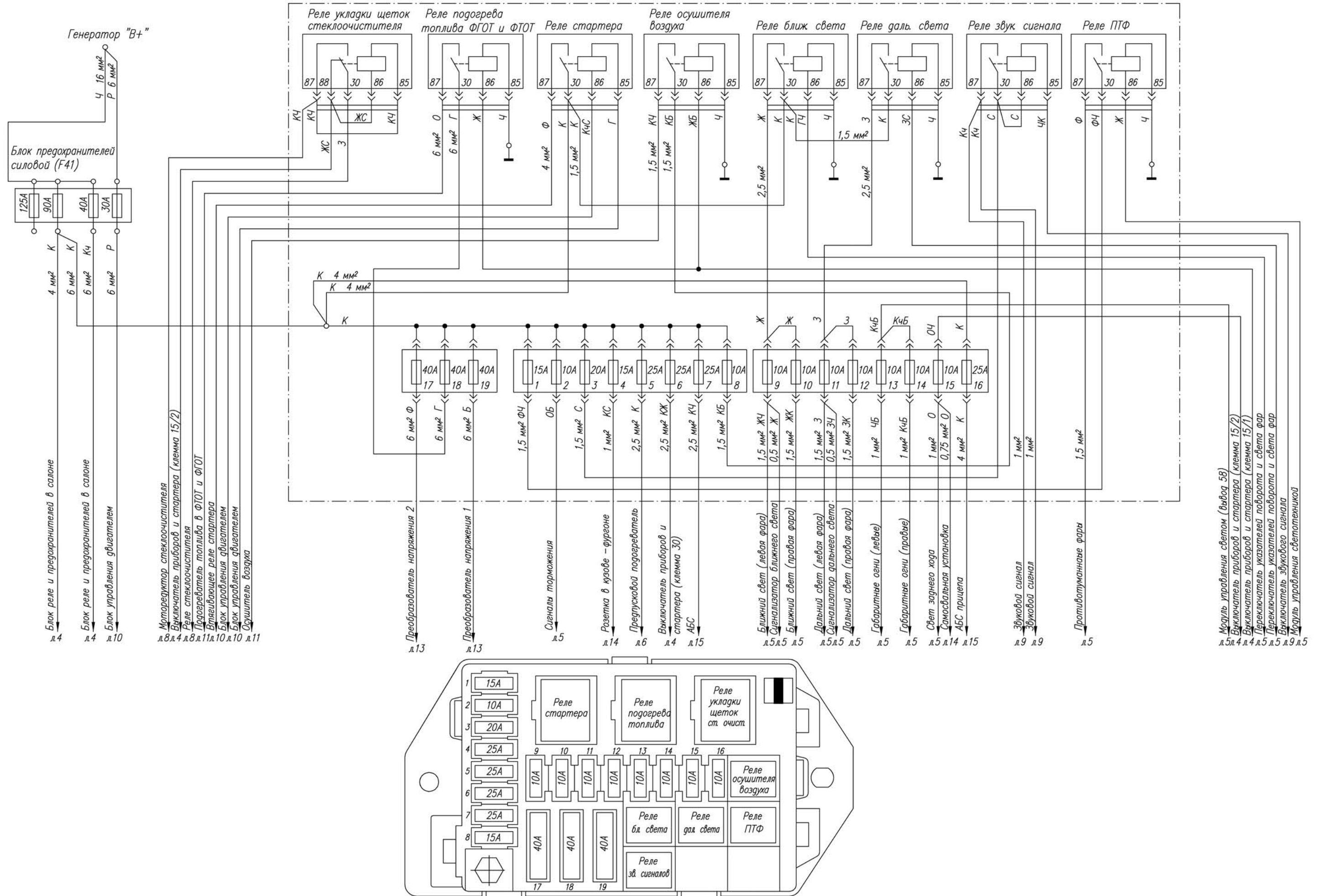
Блок реле и предохранителей под капотом (F44)
